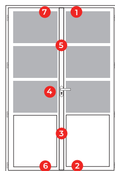
PORTE-FENÊTRE ARCAD'LUX AVEC OPTION SERRURE *
